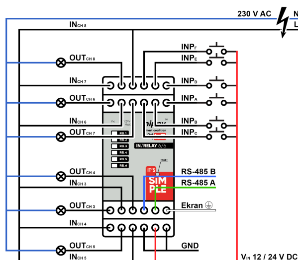
Schemat wyprowadzeń modułu nippy™ SIMPLE In/Relay 6/6 dot. sterowania wej. 12/24V DC i wyjściami przekaźnikowymi (rys.3)
