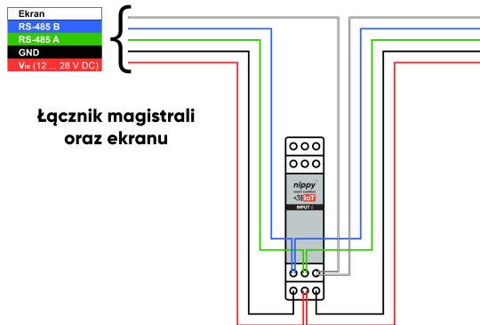
Schemat podłączenia modułu nippy™ DIN Input 6 jako łącznika magistrali oraz ekranu (rys.5)
