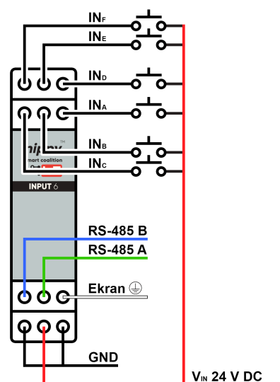
Schemat wyprowadzeń modułu nippy™ DIN Input 6 (rys.2)
