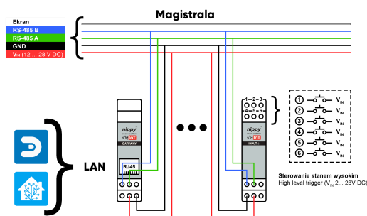
Uproszczony schemat połączeń Smart Home nippy™ z modulem nippy™ DIN Input 6 (rys.1)
