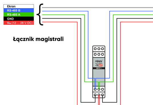
Schemat podłączenia modułu nippy™ DIN Input 6 jako łącznika magistrali (rys.4)
