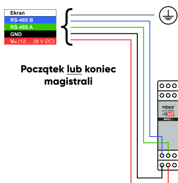
Schemat podłączenia modułu nippy™ DIN Input 6 na początku lub końcu magistrali (rys.3)
